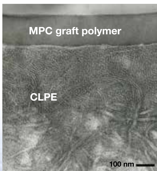
図3. MPCポリマー層の断面透過電子顕微鏡(TEM)写真
