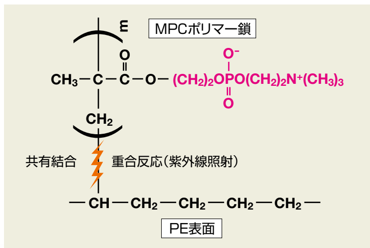
図2. 光開始ラジカルグラフト重合法の模式図
