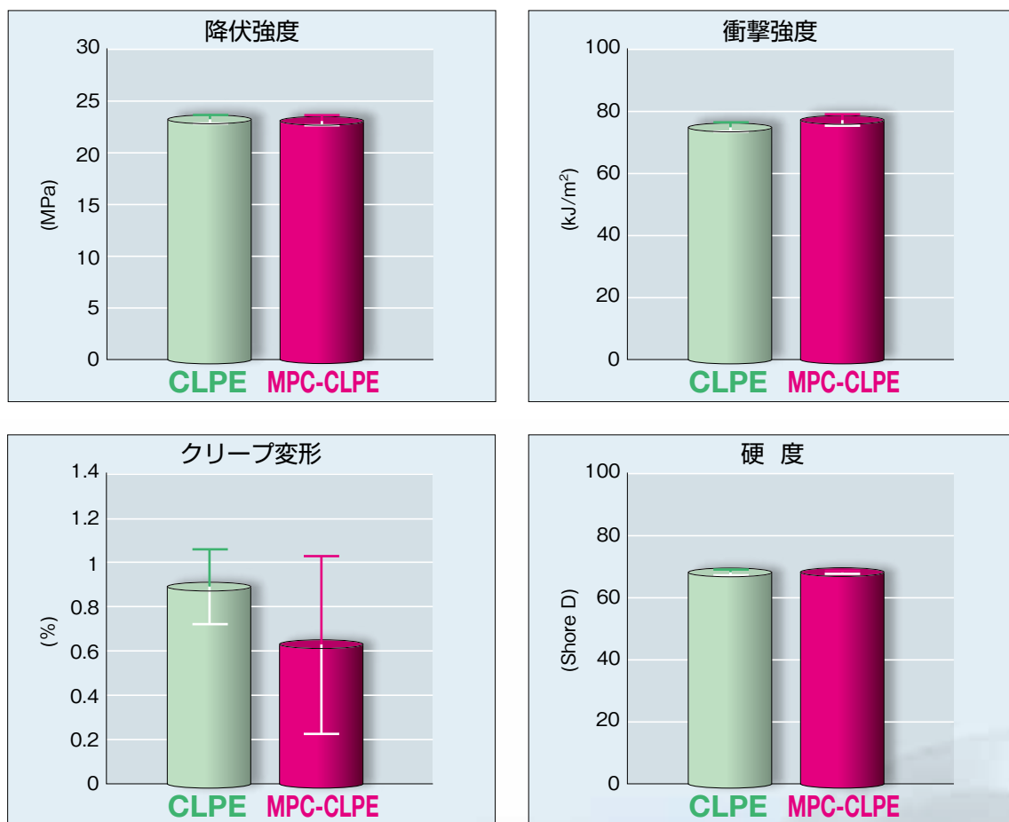
図8. Aqualaによる機械的特性の変化
