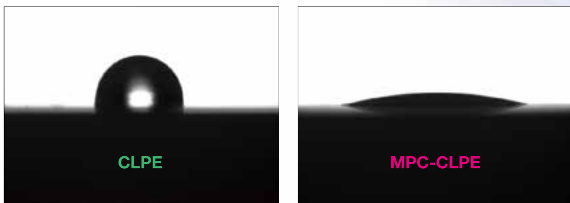
図4. 水ぬれ性の比較
