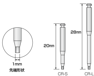
ドライバー先端形状 ■
