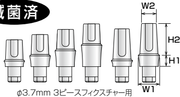
φ3.7mm 3ピースフィクスチャー用
