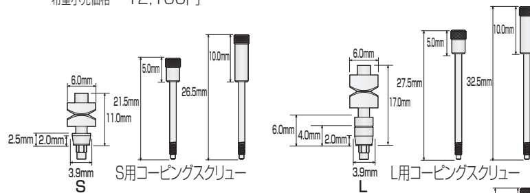
φ3.4mmフィクスチャー用 (ライトブルー)
