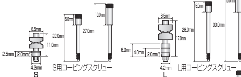
φ3.7mmフィクスチャー用 (ピンク)
