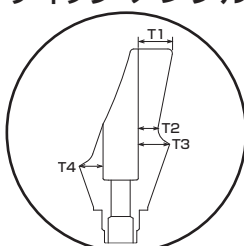
断面図
