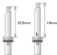
シャフト寸法
