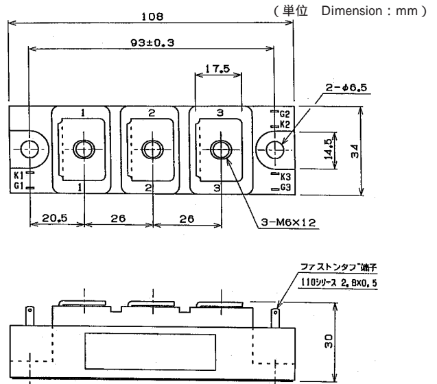
外形寸法図 OUTLINE DRAWING
