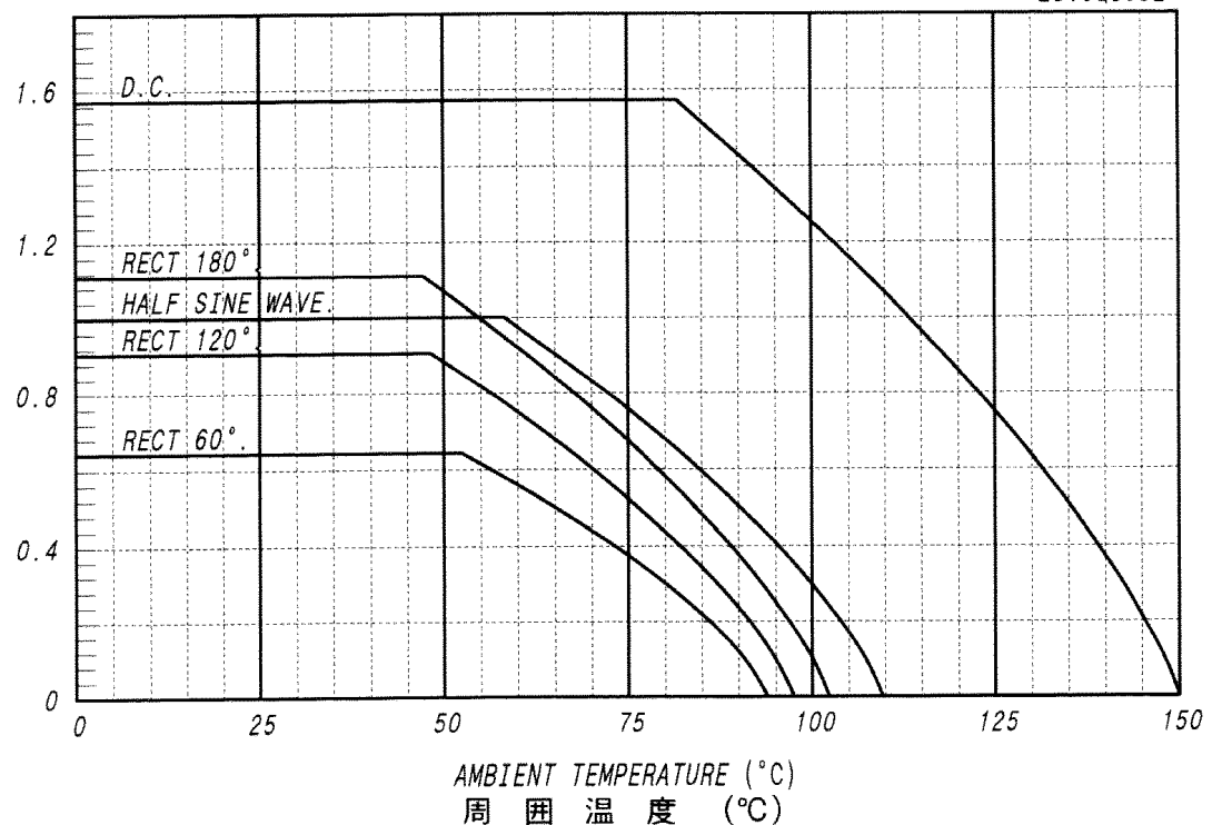
平均順電流 - 周圍溫度定格 AVERAGE FORWARD CURRENT VS. AMBIENT TEMPERATURE
